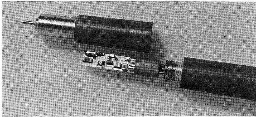
Bild 2-1 Tastkopf mit abgeschraubter Tastkopfspitze Fig. 2-1 Probe with tip screwed off
